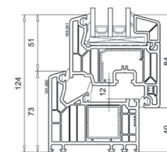
VIGO 82 (MD)
