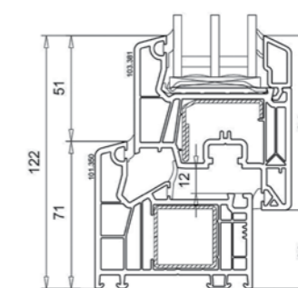
INEO 76 (MD)
